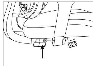
Rechten Hebel anheben, um die Sitzhöhe einzustellen.
