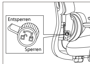
Zurücklehnen und Knopf zur Lendenstütze drehen.
