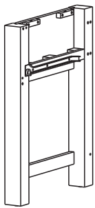
B. Side Frame 1 pc.
