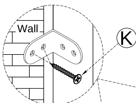
STEP 19-3: ÉTAPE 19-3:
