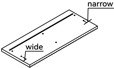
⑮(479.5x195x15mm)X1
