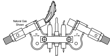
Figura 25 - Patrón incorrecto de la llama del piloto (gas natural)
