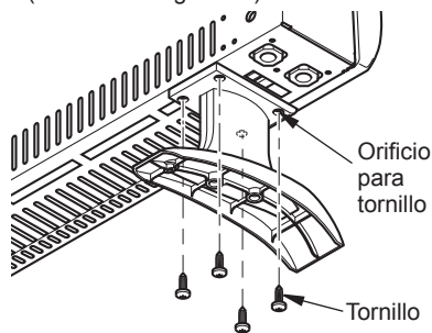
Figura 12 - Colocación de las patas de base al calentador
