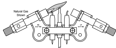
Figura 24 - Patrón correcto de la llama del piloto (gas natural)
