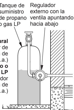
Figura 17 - Regulador externo con la ventila apuntando hacia abajo (sólo propano y gas LP)
