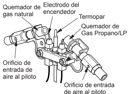
Figura 22 - Orificio de entrada de aire al piloto
