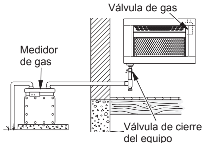
Figura 20 - Suministro de gas natural
