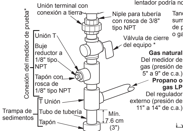
Figura 16 - Conexión de gas
