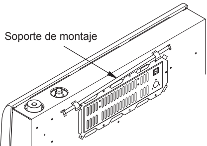
Figura 6 - Ubicación del soporte de montaje
