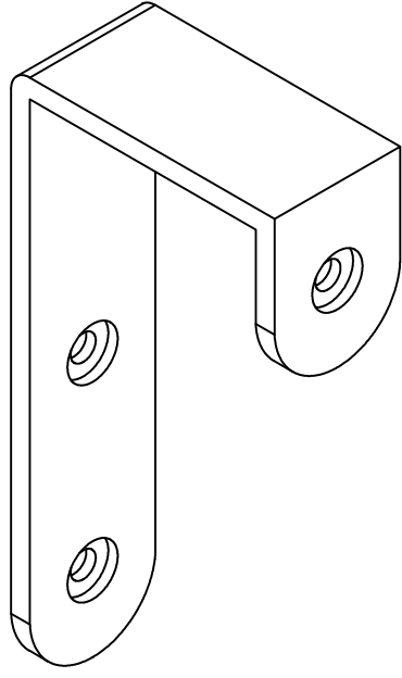
20621 (85mm*42mm*21mm)
