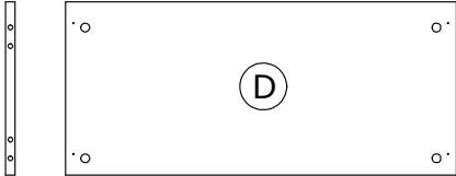
● PI4311 668x297x16mm
