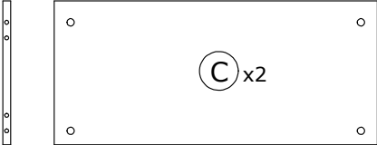
● PI4315 668x297x16mm
