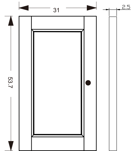
DOOR DETAIL
