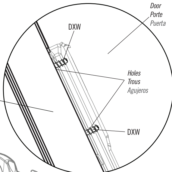
Rear of Door / La partie arrière de la porte La parte trasera de la puerta
