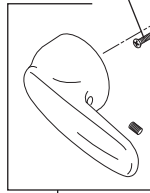
RP104450▲ Handle & Set screw Manija en Palanca y Tornillo de Ajust Manette et Vis de Calage
