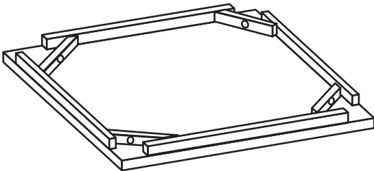
1x Table top
