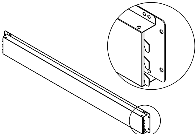
H:Bottom door frame
