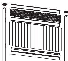
Paneles con enrejado superior
