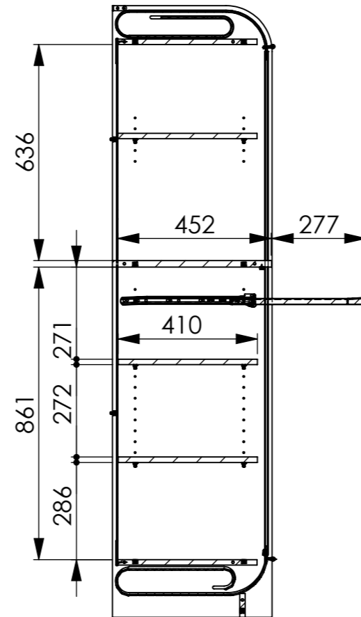
COUPE A-A ECHELLE 1 : 15.5
