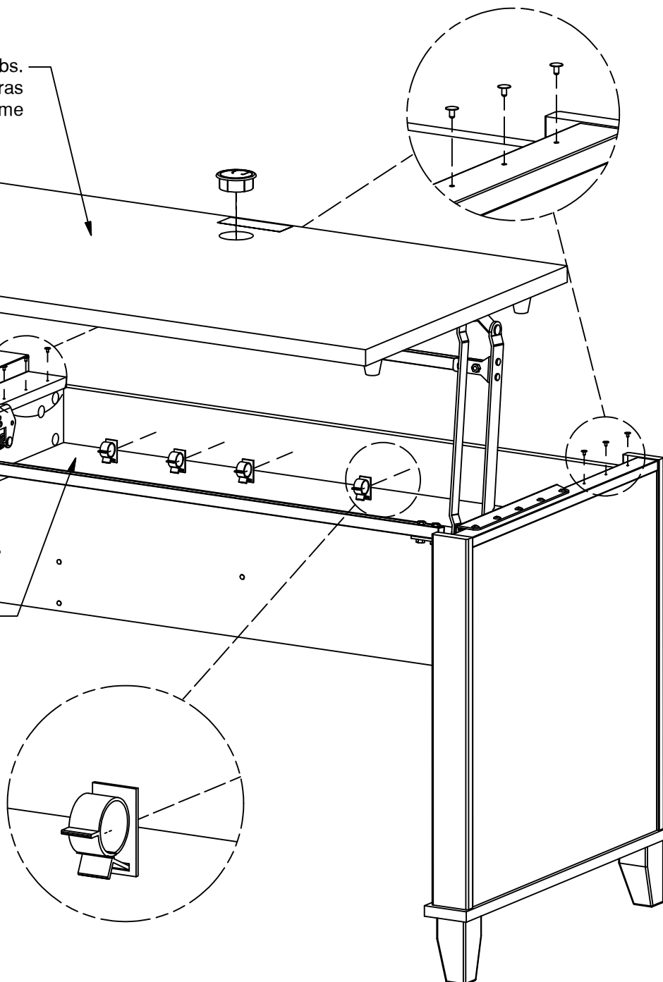
Wire Clip
