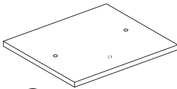
D 450*300*12mm(1pc)
