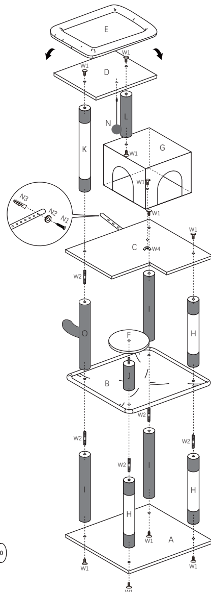
O 400*53.5mm(1pc)
