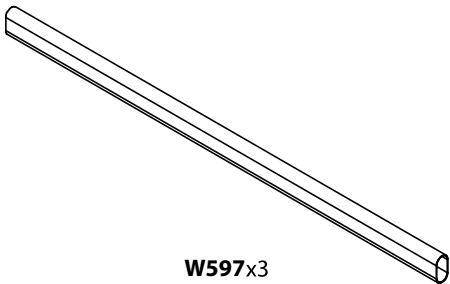
W597 x3 L. 764mm
