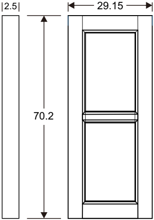
DOOR DETAIL
