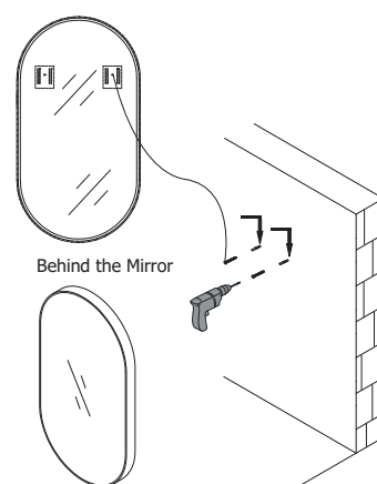
3. Hang the mirror Accrocher le miroir
