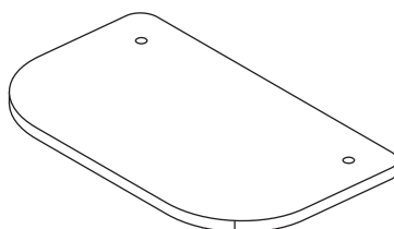
E 480*300*12mm(1pc)
