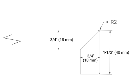
EDGE SIDE VIEW
