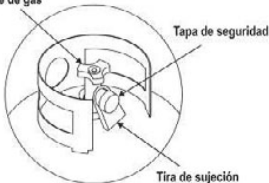
Válvula del tanque de gas
