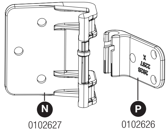
Door Hinge Charnière de porte Bisagra de la puerta x2
