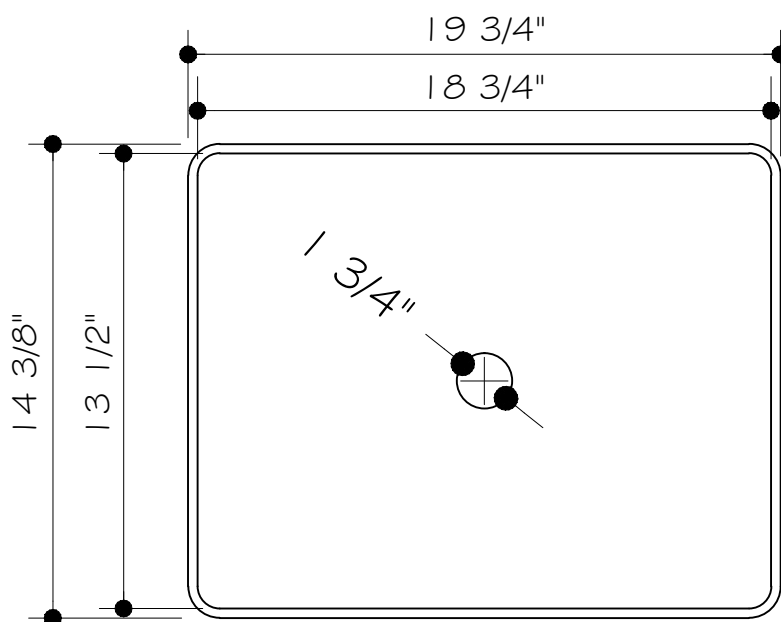
VISTA SUPERIOR
