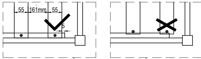
Slats distance
