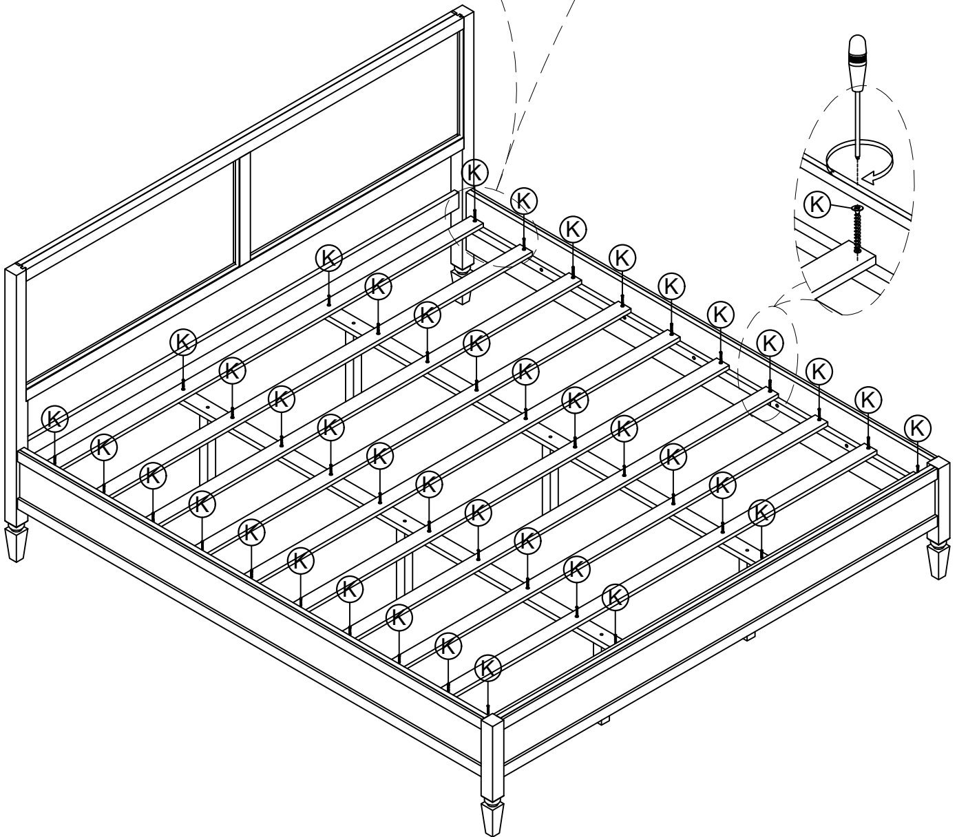
Slats distance
