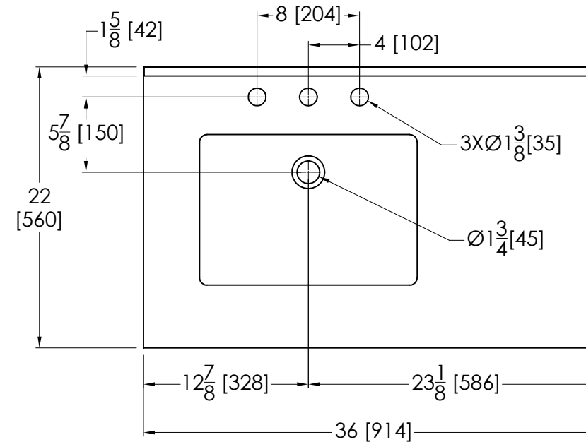
TOP / DESSUS / ARRIBA
