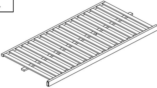
Seat Panel - 1Pc Panneau de Siège
