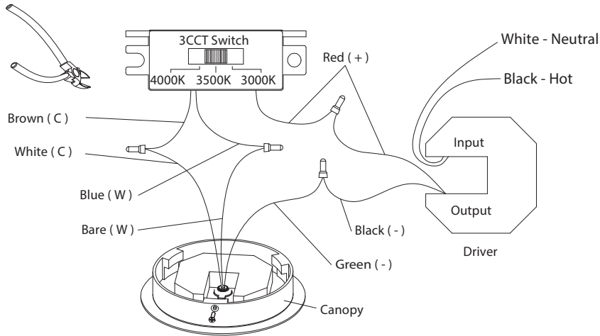
Fig. 3 Switch
