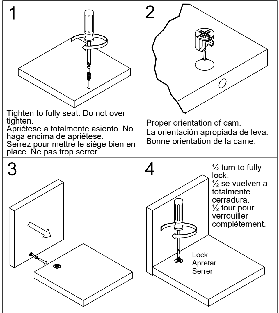
#A12210 1/2" pan head cabeza redondo 1/2" tête ronde
