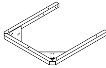
left frame*1
