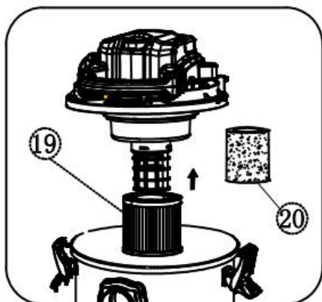
Gruppo filtro HEPA per uso a secco
