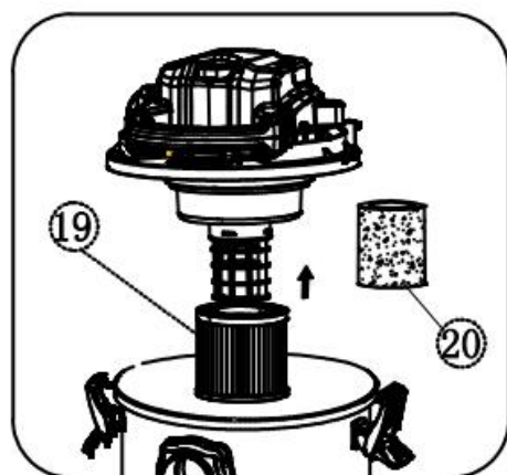
Ensemble de filtre éponge pour le nettoyage en milieu humide
