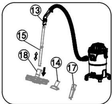
Assembler pour une utilisation sous vide
