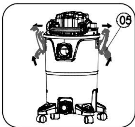
Verwendung des Laufclips
