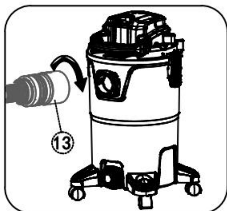
Sposób działania zespołu węża Funkcja czyszczenia
