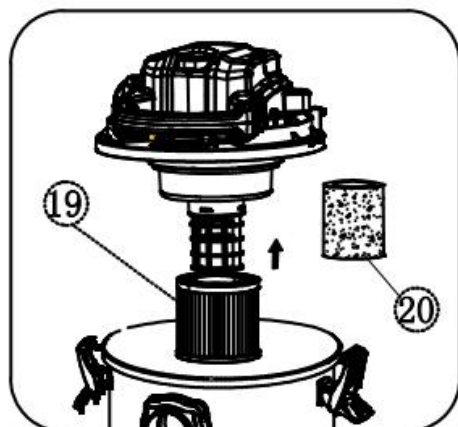
HEPA-filtermontage voor droog gebruik
