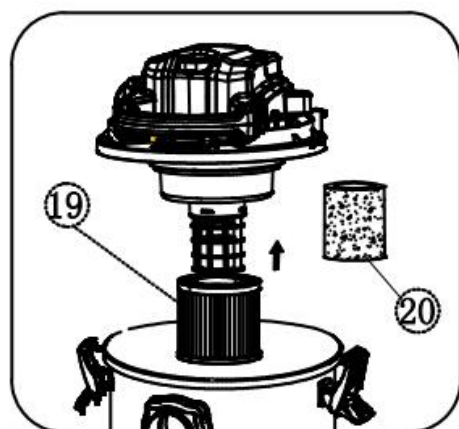
Conjunto de filtro de esponja para función de limpieza en húmedo
