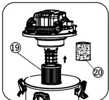
Svampfilterenhet för våtrengöring Funktion
