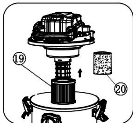
Gruppo filtro spugna per la pulizia a umido Funzione
