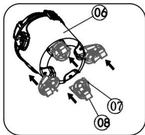
Ensamblaje de ruedas
