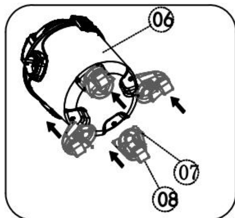
Hjulmontering
