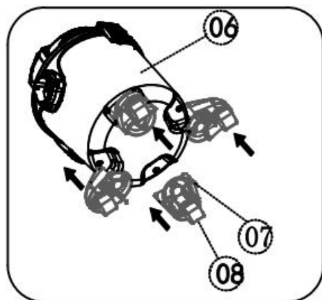
assemblage des roues
