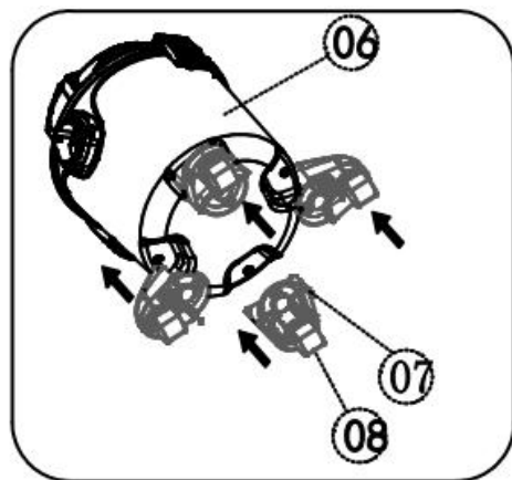
Radmontage
