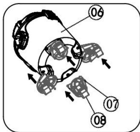
Montaż kół
