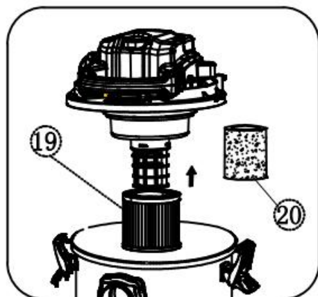
Ensemble de filtre HEPA pour usage à sec
