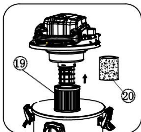
HEPA-Filterbaugruppe für den Trockenbetrieb
