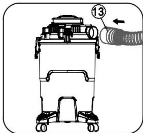
Assembler le tuyau pour le SOUFFLAGE.
