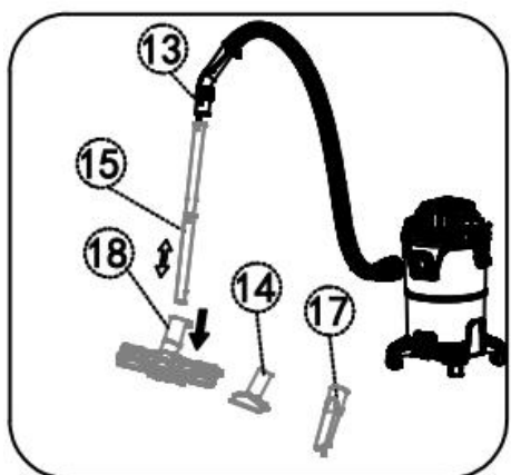
Monteren voor vacuümgebruik
