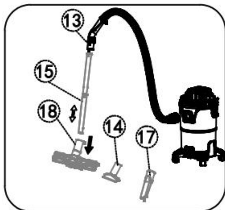
Monteras för vakuumanvändning
