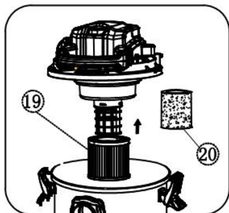
HEPA-filterenhet för torr användning
