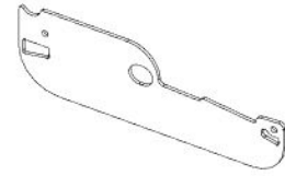
L03 LOUVER SIDE PLATE - A4M04138 (x54) 1/16"x2 3/16"x6 9/16" (2x55x167)
