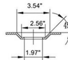
A-A 4:1
