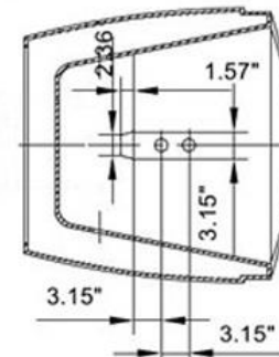
B2-B2
