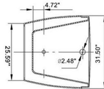
B1-B1
