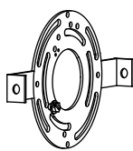
Plaque de montage (A)
