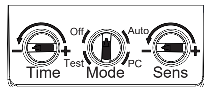
Fig. 5 (Vue de l'arrière de la lentille du détecteur)
