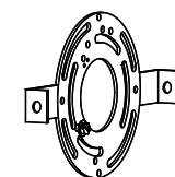
Unidad de placa de montaje (A)
