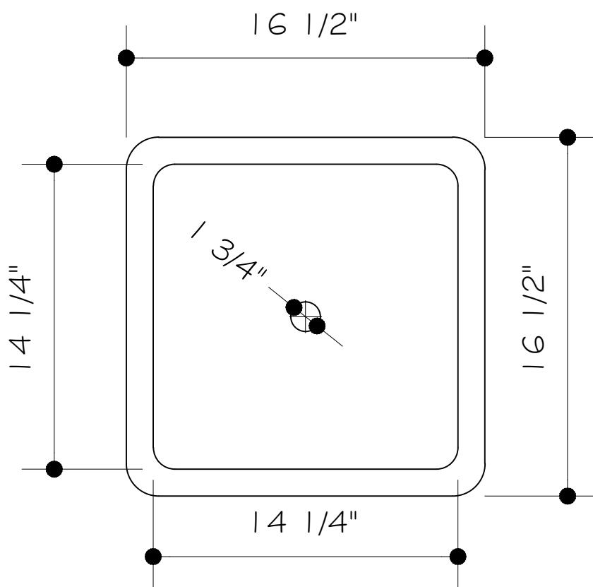
VISTA SUPERIOR
