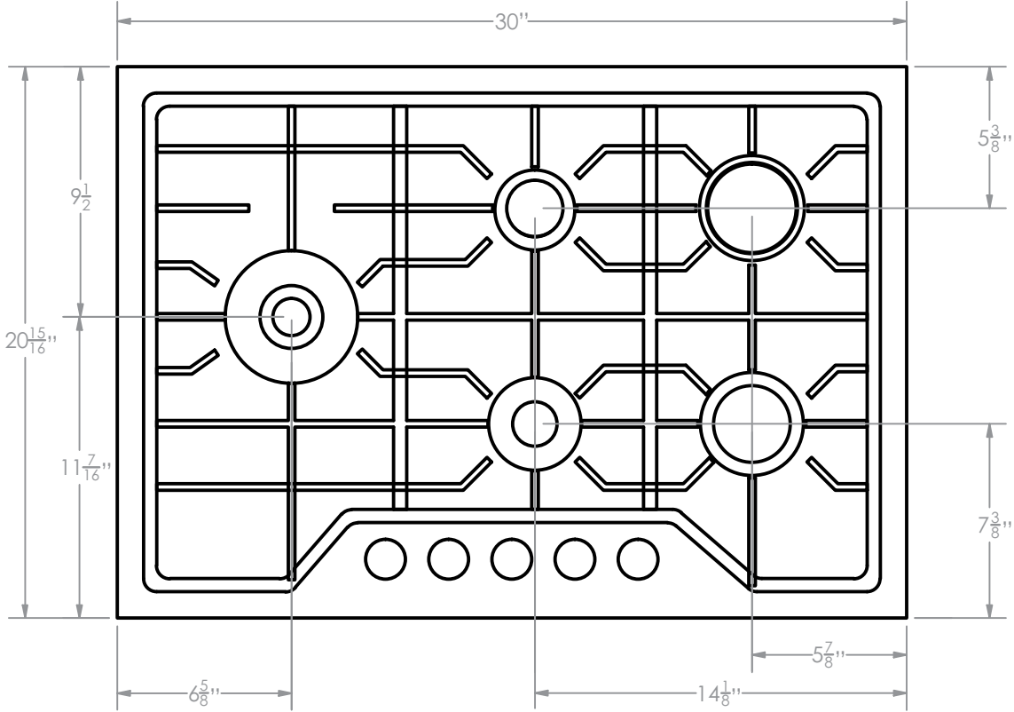
TOP
