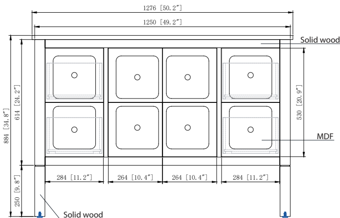
Front / Devant
