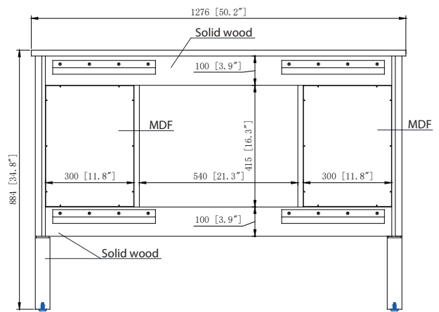
Back / Derrière
