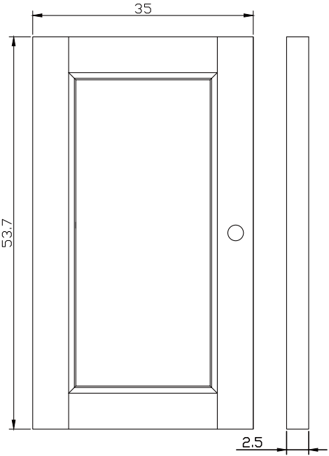
DETAIL DOOR
