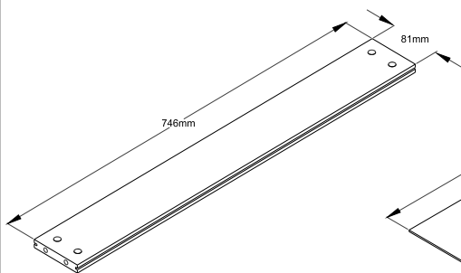
Wood Strip Qty:1
