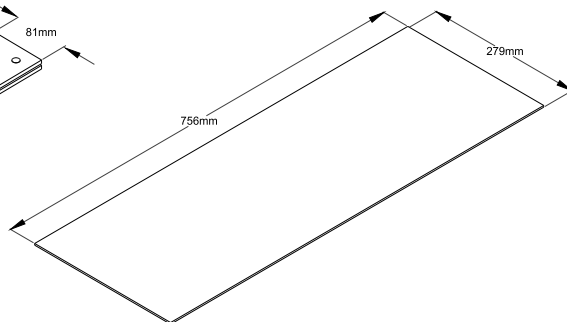
Back Panel Qty:1
