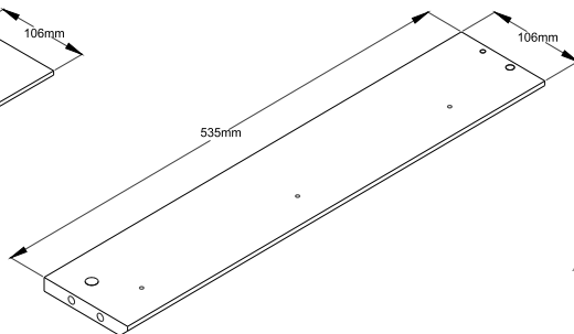
Bottom Right Brace Panel Qty:1
