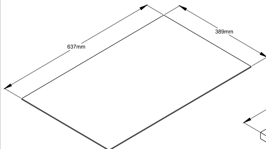
Drawer Bottom Panel Qty:2
