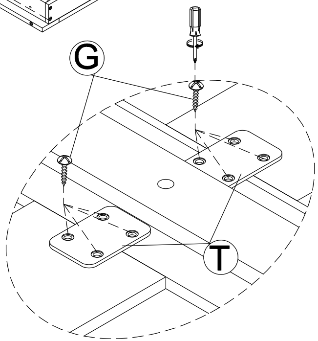
Detail 2(x2) Détail 2(x2)
