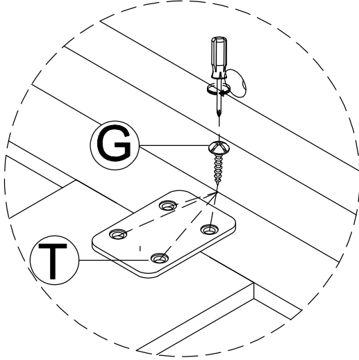
Detail 1(x2) Détail 1(x2)
