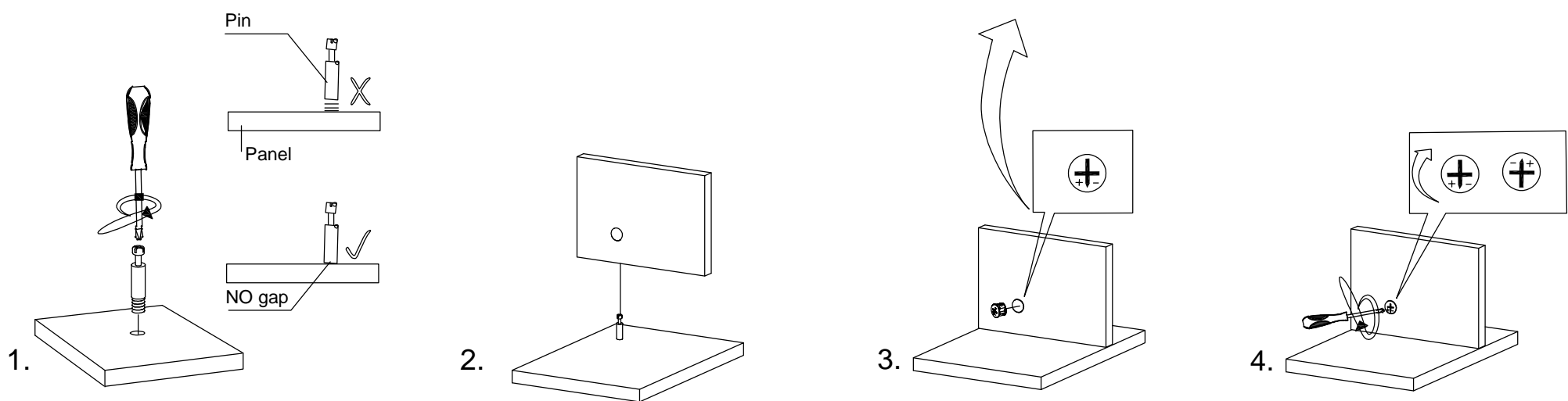
Bolt
