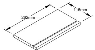
DRAWER BACK Qty:1
