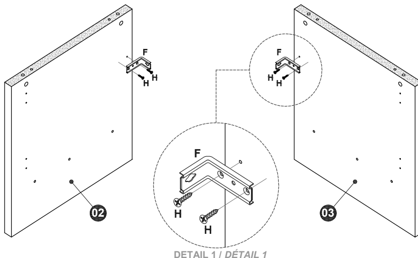
DETAIL 1 / DÉTAIL 1
