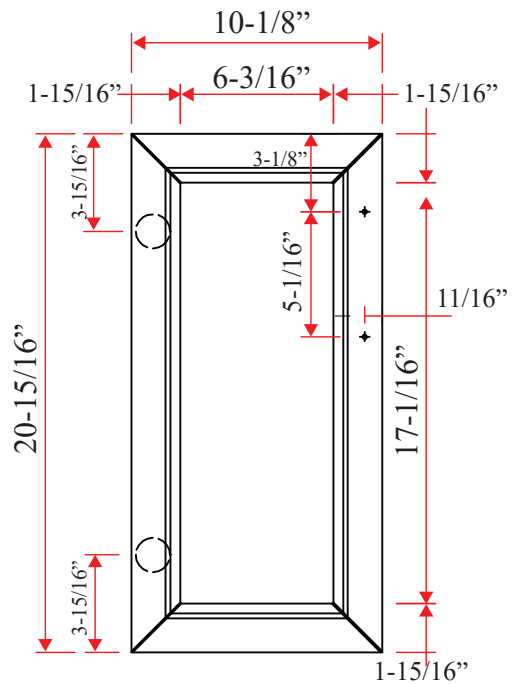
— DOOR PANEL —
