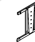
(A) Left leg Pata izquierda 1 part/pieza
