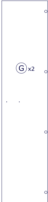
● AN1939 2039x465x16mm
