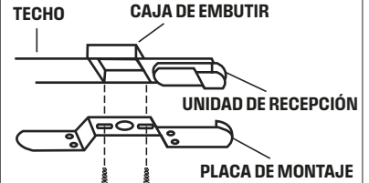
FIGURE - 5 SÓLO VENTILADORES DE MONTAJE ALTECHO
