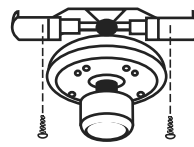
FIGURE - 4 SÓLO VENTILADORES CON VARILLA VERTICAL
