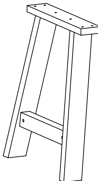
LEG (L&R Same) QTY 2
