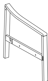
Armrest
