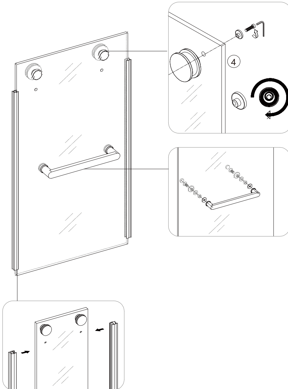
Door Glass
